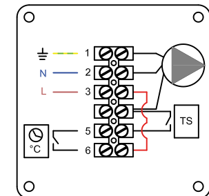
Подключение к комнатному термостату Connection with room thermostat
