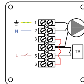
Прямое соединение с переключателем Direct connection with switch
